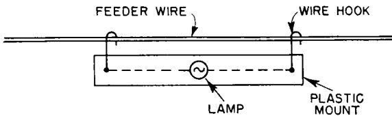
FIG. 4.61. Miniature-lamp indicator.
